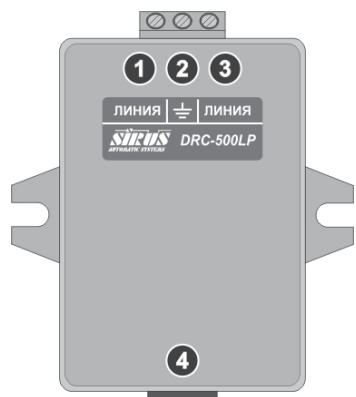
Рисунок 7. Внешний вид Устройства Защиты Линии SIRUS DRC-500LP
